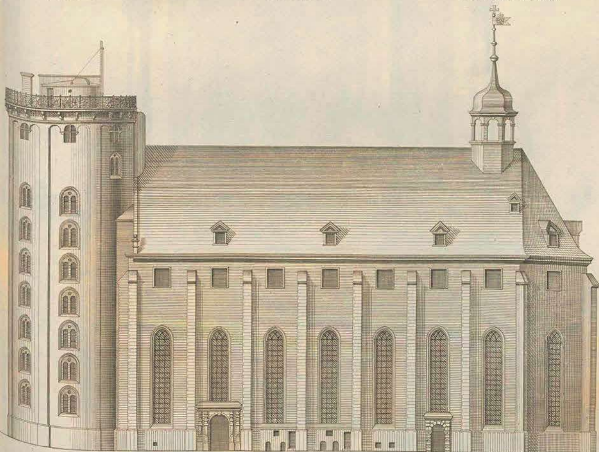
Giennem-Snitt eller Profil af Trinitatis Kirke
