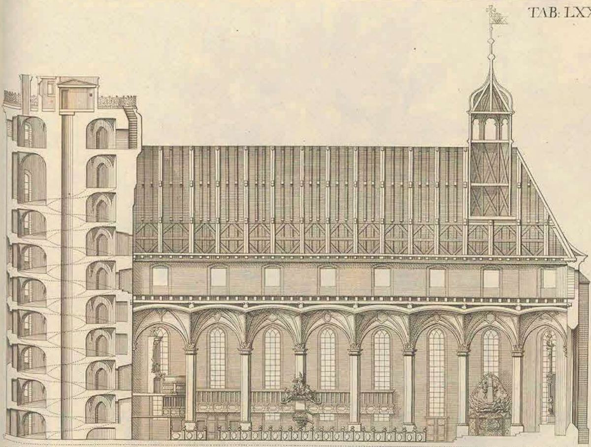
Coupe ou Profil de l'Eglise de la Trinite.
